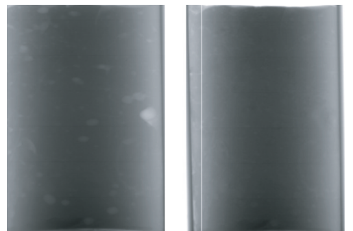
(a) 共振声混合工艺 (b) 现有混合工艺 图5 PBX-X炸药不同混合工艺CT照片
