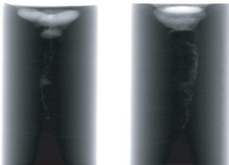
(a) 共振声混合工艺 (b) 搅拌混合工艺 图3 B炸药不同混合工艺CT照片
