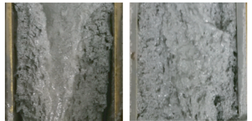
(a) 共振声混合工艺 (b) 现有混合工艺 图4 PBX-X炸药药浆照片
