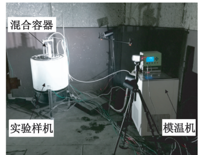
图 1 实验现场设备
